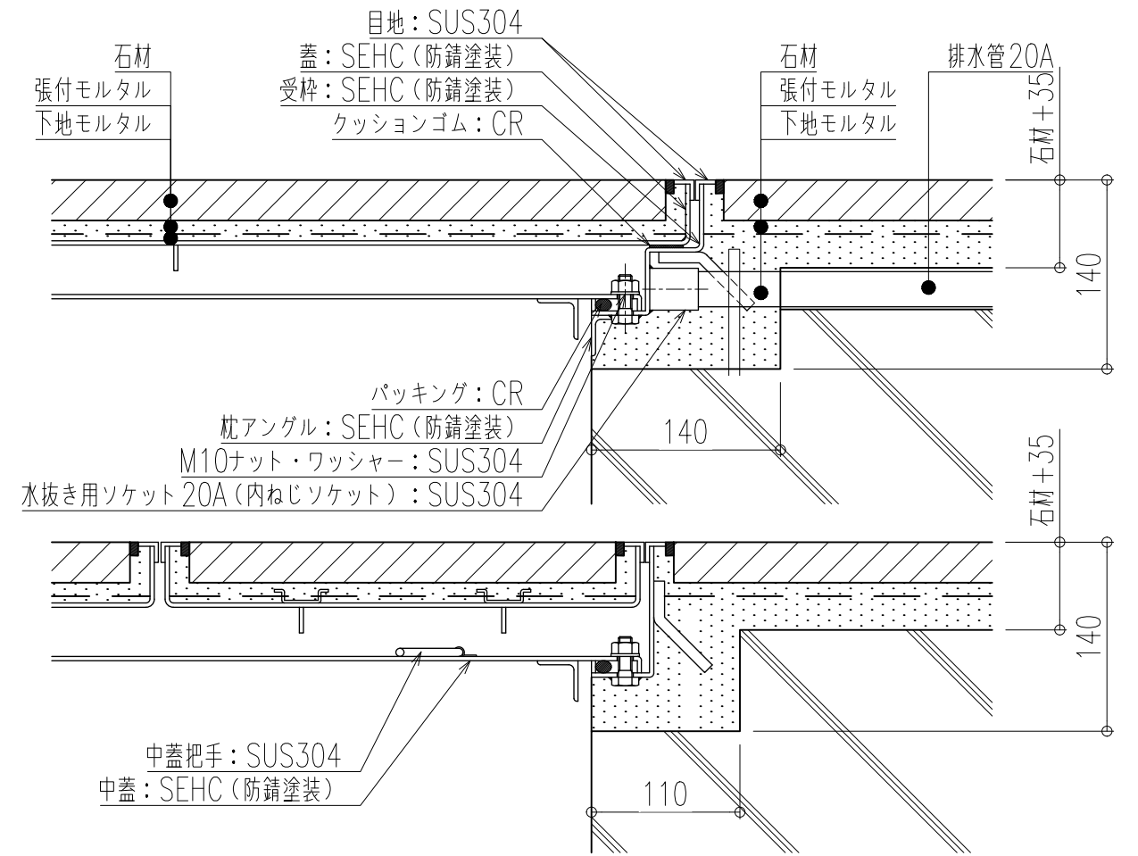
施工参考拡大図
