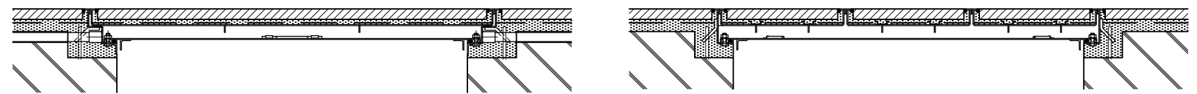
施工参考図
